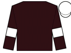
CUMULONIMBUS
